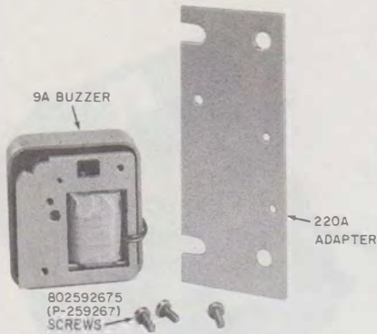
Fig. 5—9C Buzzer
