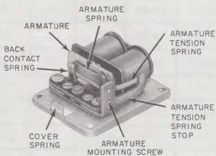
Fig. 1—7F Buzzer
