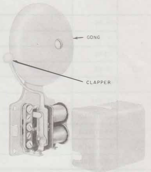
Fig. 2—7-Type Bell
