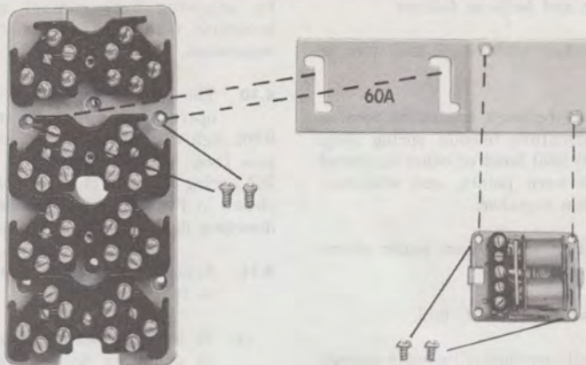
Fig. 16—60A Bracket
