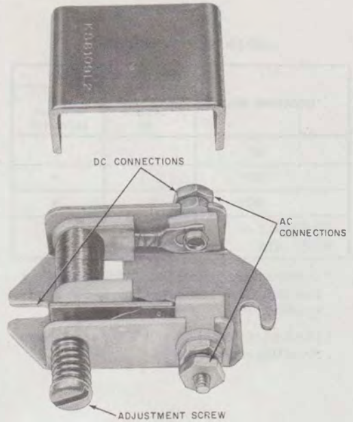
Fig. 6—KS-8109L2 Buzzer
