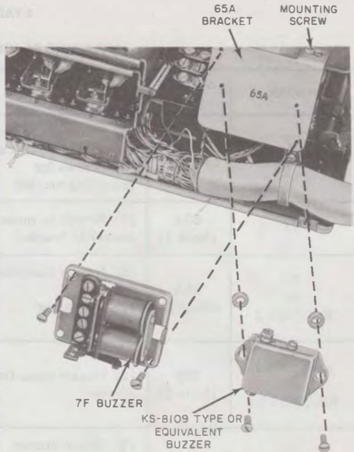
Fig. 14—65A Bracket
