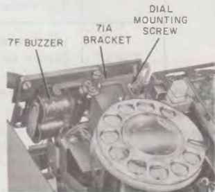
Fig. 15—71A Bracket
