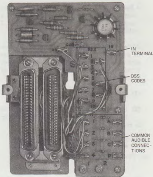
Fig. 17—25A Apparatus Unit Base
